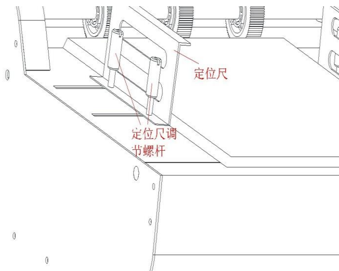
Боковые упоры
